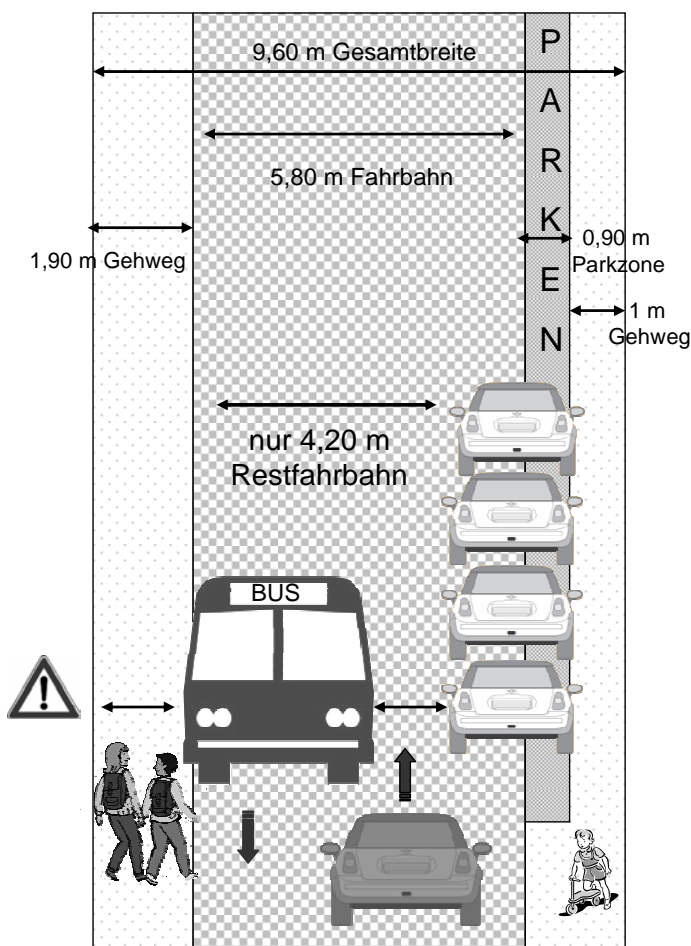
ungelöste Verkehrskonflikte Berliner Str. – gefährlicher Engpass (siehe auch Foto re. oben)
